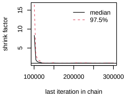
d.Erlotinib.Erlotinib_Autophagy
