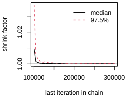
d.Erlotinib.Erlotinib_antiangio
