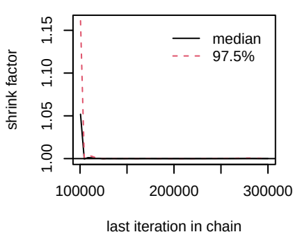
d.Gefitinib.Gefitinib_chemo
