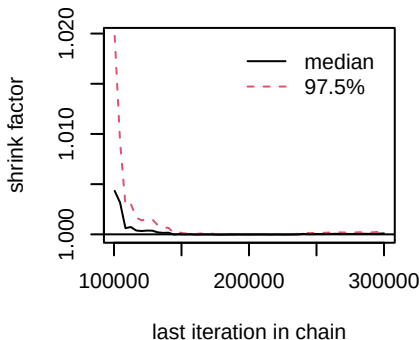
d.Afatinib.Afatinib_Cetuximab
