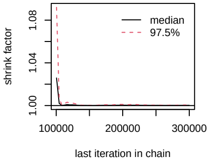
d.chemo.Erlotinib
