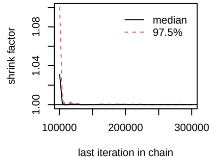
d.chemo.Osimertinib
