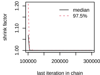
d.Erlotinib.Erlotinib_chemo
