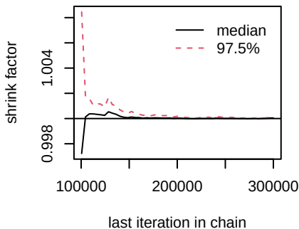
d.Erlotinib.antiangi
