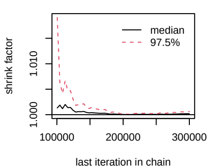
d.Afatinib.Placebo
