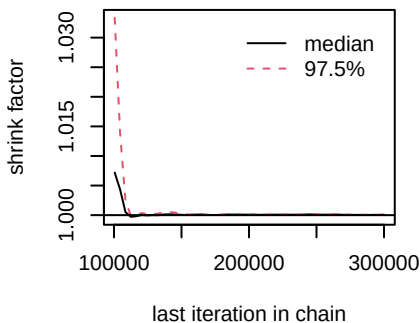
d.Osimertinib.Gefitinib_Erlotinibd.Osimertinib.Lazertinib_Amivanta d.Osimertinib.Osimertinib_antiang
