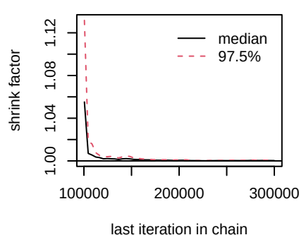
d.Erlotinib.Rociletinib
