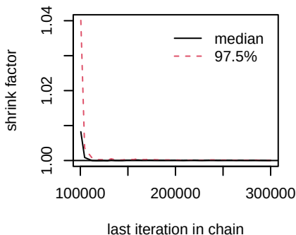
d.Erlotinib.Erlotinib_MMPI
