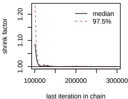
d.Erlotinib.Erlotinib_HGFi
