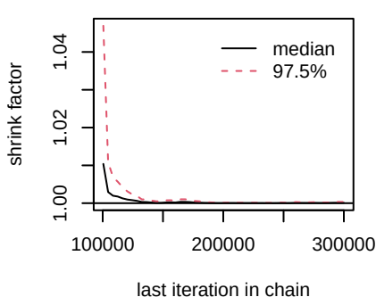
d.Erlotinib.Gefitinib_ERI
