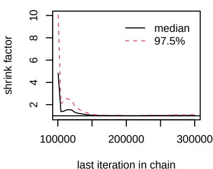
d.Gefitinib.Almonertinib
