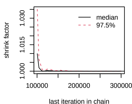
d.Gefitinib.Lazertinib
