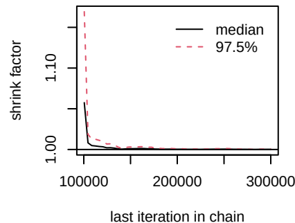
d.Erlotinib.DHFRi
