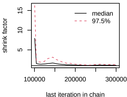
d.Erlotinib.Erlotinib_COX2i
