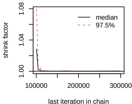
d.Erlotinib.Erlotinib_ERi
